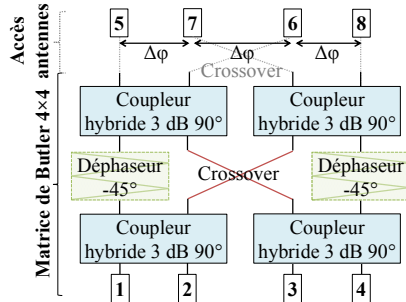
Figure 1. Diagramme d'une matrice de Butler 4×4.
