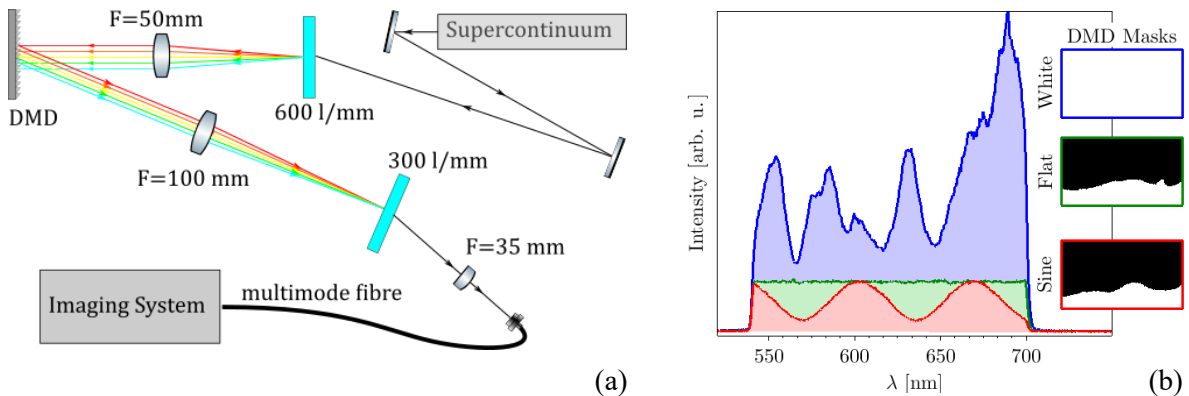
Fig. 1 : (a) Schéma du design de la source structurable spectralement; (b) Exemple de spectres générés par le système avec leur masque respectif.
