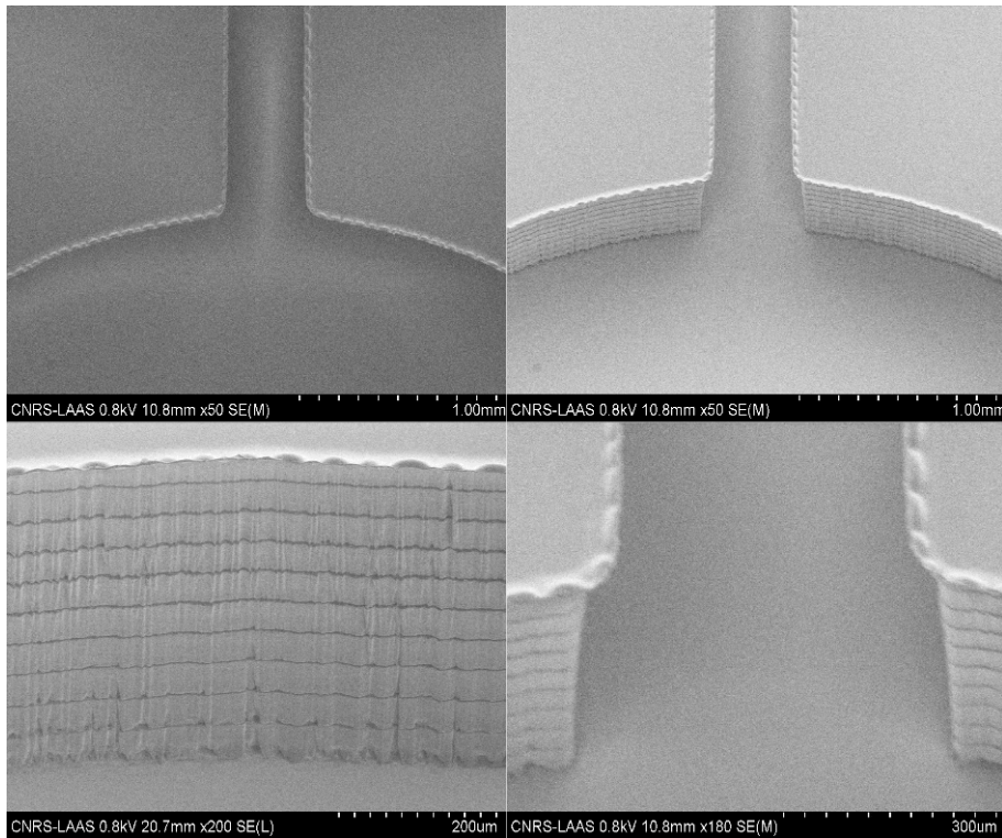
FIGURE 3.41 – Images MEB des biopuces DF/Verre
